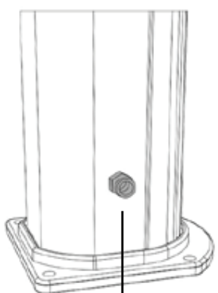
Alimentazione 1/2' Water supply 1/2'
